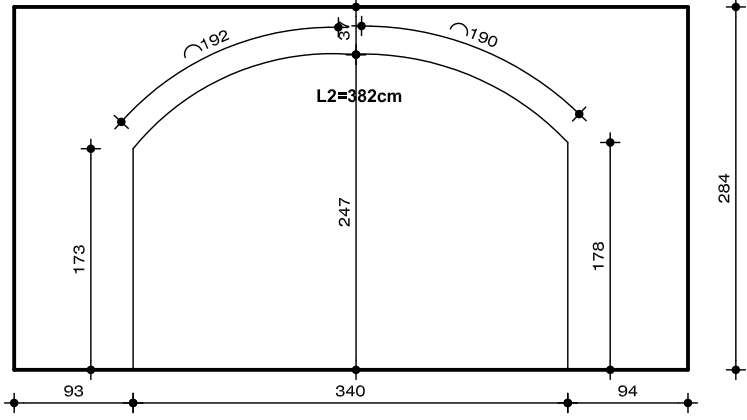
PRESEK D-D
